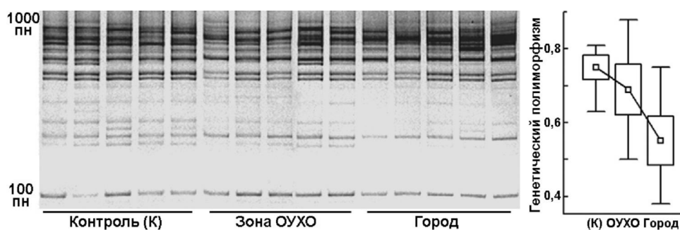
Рис. 10. Электрофореграмма фрагментов амплификации с RAPD-праймером ОРА-01 (слева) и уровень генетического полиморфизма (справа) экземпляров озерной лягушки из трех исследованных биотопов с разной антропогенной нагрузкой
