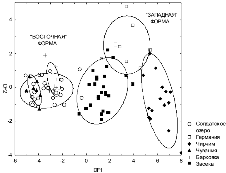
Рис. 7. Распределение параметров звуковых сигналов озерной лягушки из шести популяций в пространстве двух первых дискриминантных функций
