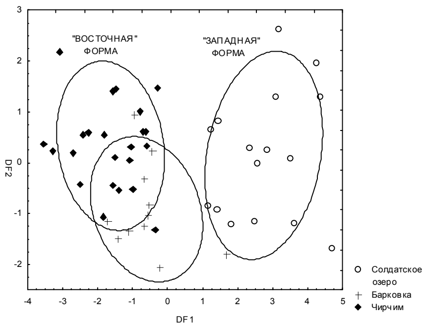
Рис. 6. Распределение морфометрических индексов озерной лягушки из трех популяций в пространстве двух дискриминантных функций
